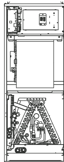
Fig. 12 — Air Handler
