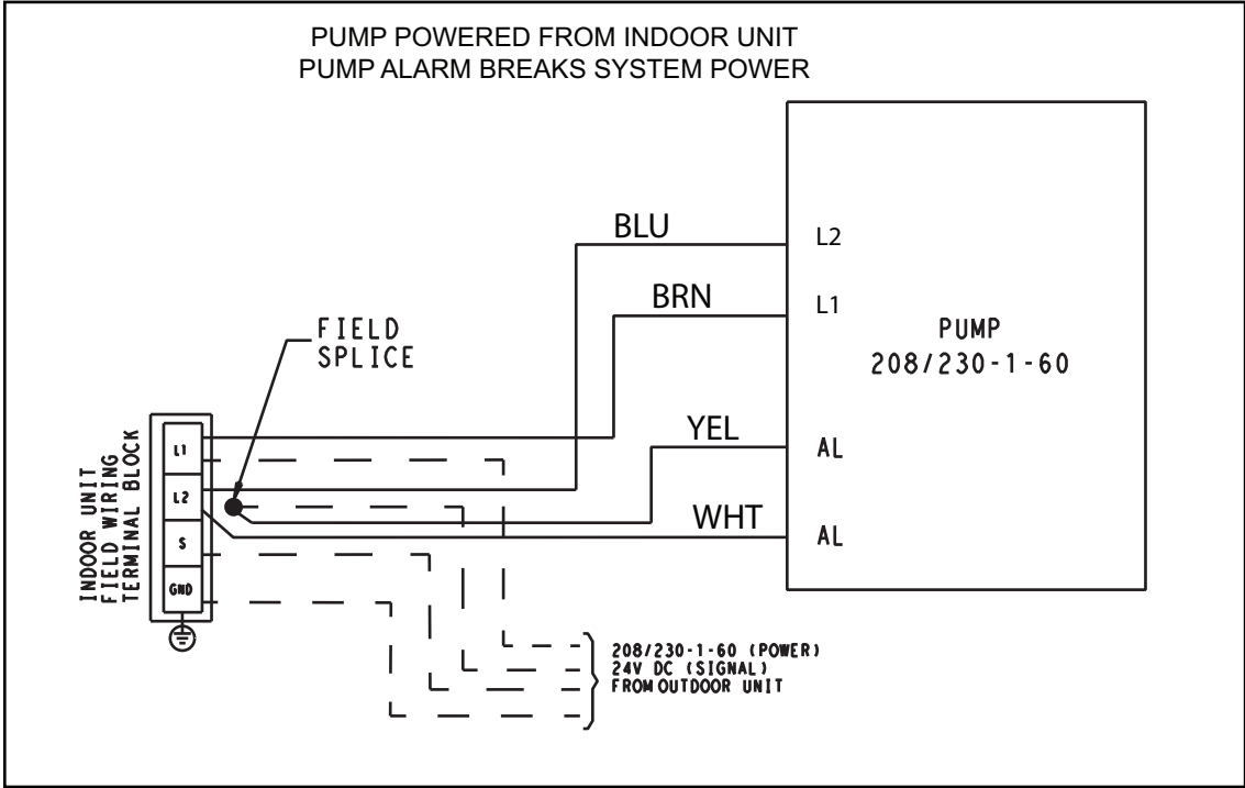
Fig. 13 - (208/230-1-60) WIRING SCHEMATIC
