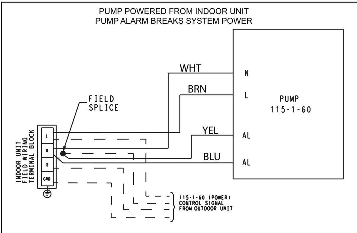
Fig. 11 – (115-1-60) WIRING SCHEMATIC
