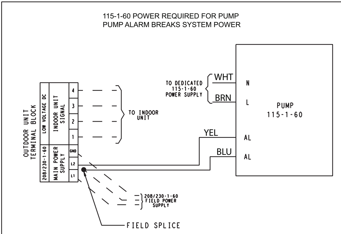
Fig. 10 – (115-1-60) WIRING SCHEMATIC
