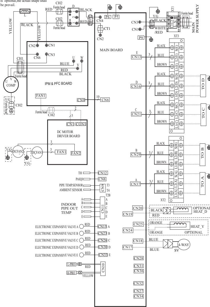
Fig. 15 – Wiring Diagrams 36K – 4 Zone Max
