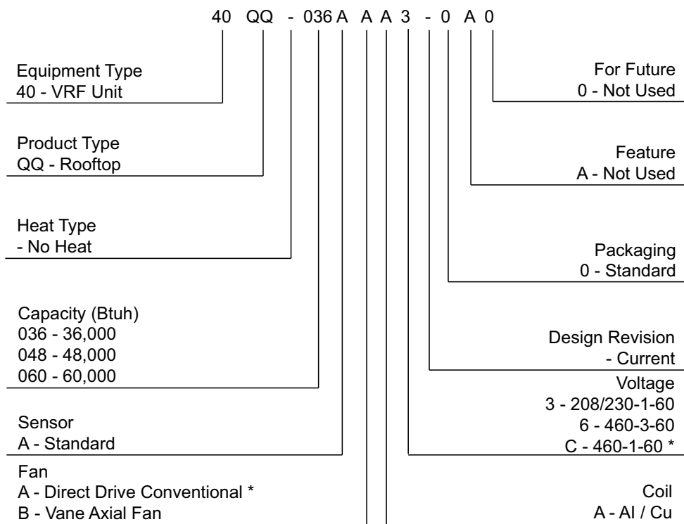
Fig. 1 —Nomenclature
