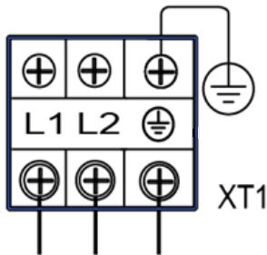
Fig. 4 —Power Input
