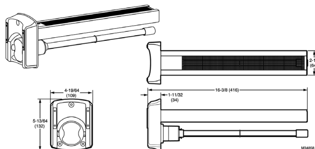
Fig. 1. UV2400U5000, Dimensions en po (mm).
